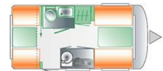
Wohnwagen Eifelland 395
